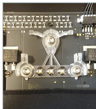
Źródło światła Futurled6-300mm zainstalowane w obudowie (NOWE)
