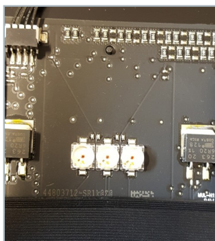
Źródło światła Futurled3R-300mm zainstalowane w obudowie (STARE)
